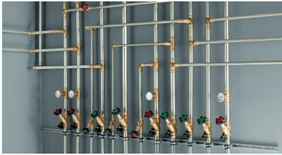
Внутренние трубопроводы
